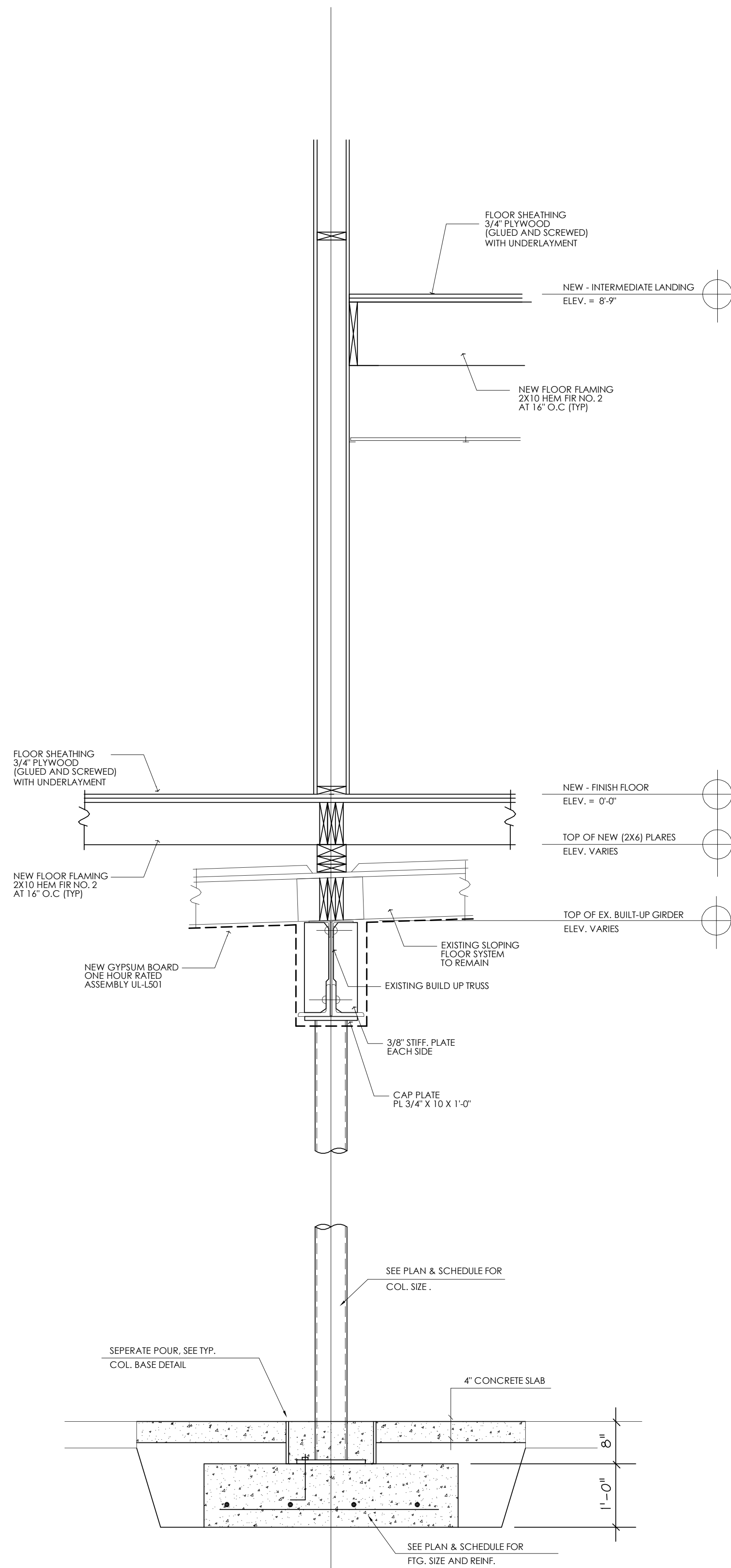
SECTION SCALE: 1/4" = 1'-0" 2 A2.1
